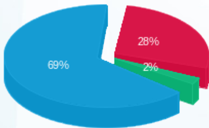
פסגה (Kwh 46,372.29) 28% גבע (Kwh 3,656.81) 2% שפל (Kwh 113,429.67) 69%
