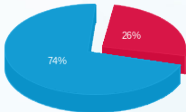
■ פסגה (Kwh 211,900.82) ■ גבע (Kwh 0.00) ■ שפל (Kwh 613,086.38)
