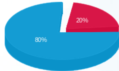
■ פסגה (67,401.40 Kwh) ■ גבע (0.00 Kwh) ■ שפל (261,528.60 Kwh)
