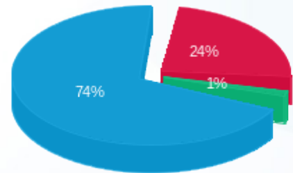
■ פסגה (25.83 Kwh) ■ גבע (1.39 Kwh) ■ שפל (78.37 Kwh)
