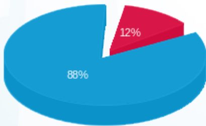
■ פסגה (5,511.03 Kwh) ■ גבע (0.00 Kwh) ■ שפל (41,305.83 Kwh)
