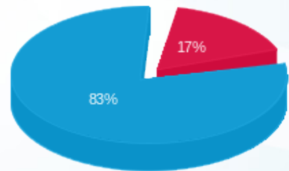
■ פסגה (243.68 Kwh) ■ גבע (0.00 Kwh) ■ שפל (1,219.80 Kwh)
