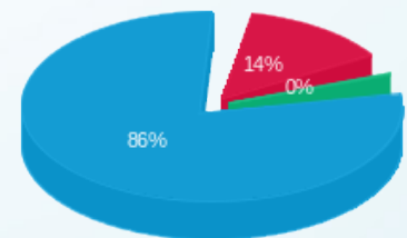
פסגה (Kwh 5,746.77) גבע (Kwh 68.03) שפל (Kwh 35,429.64)
