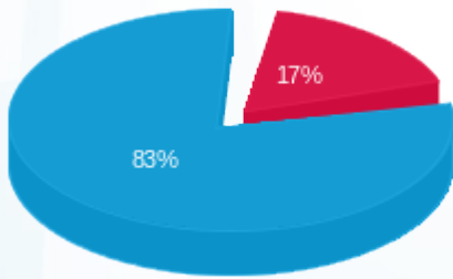
■ פסגה (Kwh 18,218.28) ■ גבע (Kwh 0.00) ■ שפל (Kwh 88,681.35)
