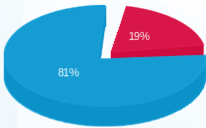
פסגה (Kwh 53,367.80) ■ גבע (Kwh 0.00) ■ שפל (Kwh 221,920.20) ■
