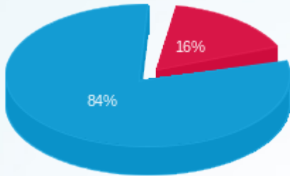
■ פסגה (40,344.19 Kwh) ■ גבע (0.00 Kwh) ■ שפל (211,060.00 Kwh)
