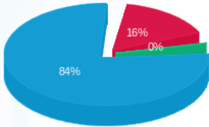
פסגה (Kwh 93,096.12) ■ גבע (Kwh 30.15) ■ שפל (Kwh 475,166.68) ■
