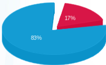
■ פסגה (30,425.62 Kwh) ■ גבע (0.00 Kwh) ■ שפל (146,716.66 Kwh)
