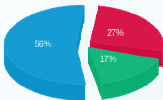
■ פסגה (Kwh 29,380.72) ■ גבע (Kwh 18,489.90) ■ שפל (Kwh 60,662.79)
