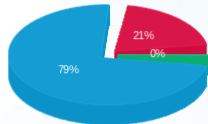
■ פסגה (Kwh 37,916.90) ■ גבע (Kwh 13.20) ■ שפל (Kwh 146,881.80)
