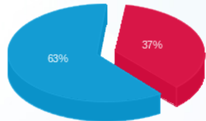
■ פסגה (17,029.57 ₪) ■ גבע (0.00 ₪) ■ שפל (29,599.76 ₪)
