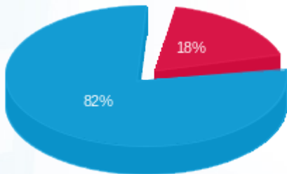
■ פסגה (16,646.70 Kwh) ■ גבע (0.00 Kwh) ■ שפל (76,643.60 Kwh)
