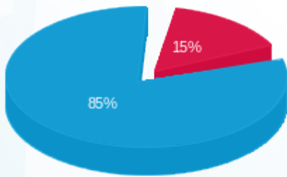
פסגה (22,541.70 Kwh) ■ גבע (0.00 Kwh) ■ שפל (126,894.43 Kwh) ■
