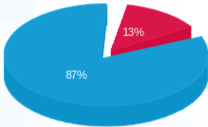
■ פסגה (13,082.95 Kwh) ■ גבע (0.00 Kwh) ■ שפל (85,348.47 Kwh)
