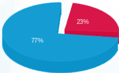
פסגה (Kwh 149,076.98) ■ גבע (Kwh 0.00) ■ שפל (Kwh 496,032.14) ■
