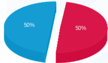
■ פסגה (Kwh 423,690.91) ■ גבע (Kwh 0.00) ■ שפל (Kwh 425,541.25)
