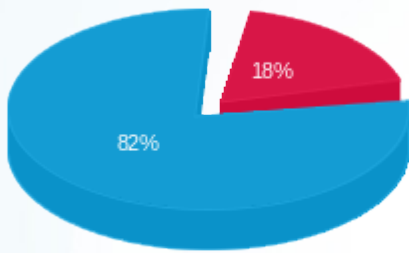
■ פסגה (84,969.28 Kwh) ■ גבע (0.00 Kwh) ■ שפל (385,648.20 Kwh)
