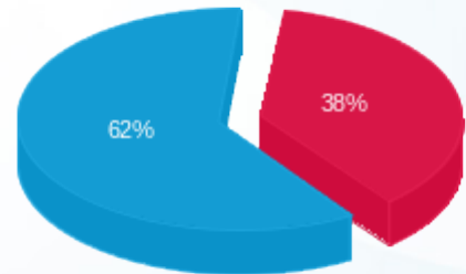
■ פסגה (666.47 Kwh) ■ גבע (0.00 Kwh) ■ שפל (1,109.62 Kwh)
