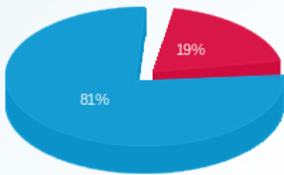
■ פסגה (80,743.20 Kwh) ■ גבע (0.00 Kwh) ■ שפל (339,935.19 Kwh)
