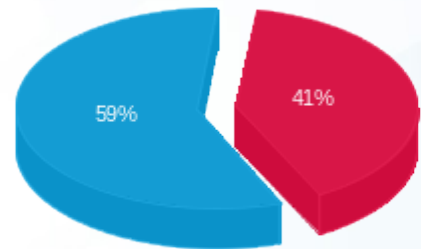
■ פסגה (14,761.82 Kwh) ■ גבע (0.00 Kwh) ■ שפל (21,298.17 Kwh)
