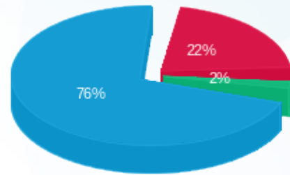
■ פסגה (Kwh 166,944.02) ■ גבע (Kwh 13,295.10) ■ שפל (Kwh 583,028.10)
