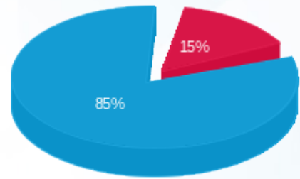
פסגה (Kwh 18,438.38) 15% גבע (Kwh 0.00) 85% שפל (Kwh 107,513.85)
