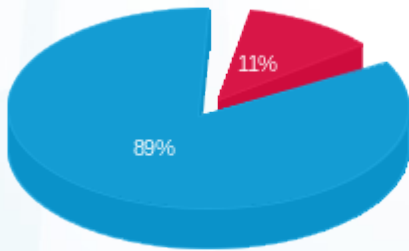
■ פסגה (17,599.17 Kwh) ■ גבע (0.00 Kwh) ■ שפל (137,713.76 Kwh)
