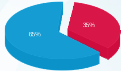
■ פסגה (7,961.34 ₪) ■ גבע (0.00 ₪) ■ שפל (15,046.22 ₪)
