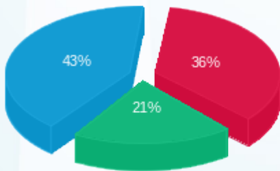
■ פסגה (65,372.40 Kwh) ■ גבע (37,276.65 Kwh) ■ שפל (76,466.59 Kwh)
