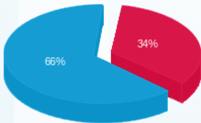
■ פסגה (3,242.68 Kwh) ■ גבע (0.00 Kwh) ■ שפל (6,248.48 Kwh)
