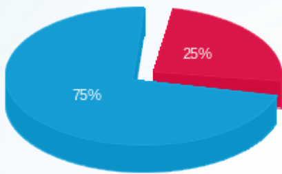
פסגה (Kwh 31,074.58) ■ גבע (Kwh 0.00) ■ שפל (Kwh 95,523.97) ■
