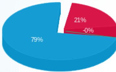
■ פסגה (284,755.83 Kwh) ■ גבע (0.002 Kwh) ■ שפל (1,094,506.13 Kwh)
