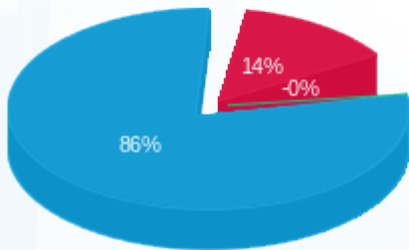
פסגה (Kwh 33,425.02) ■ גבע (Kwh -527.96) ■ שפל (Kwh 202,120.66) ■
